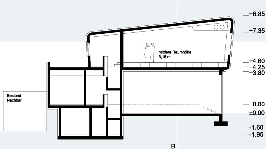
SCHNITT A
